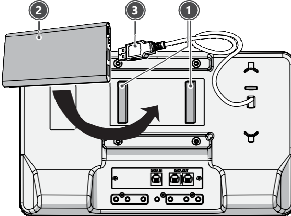
5. ábra. Tápegységgel történő tápellátás
