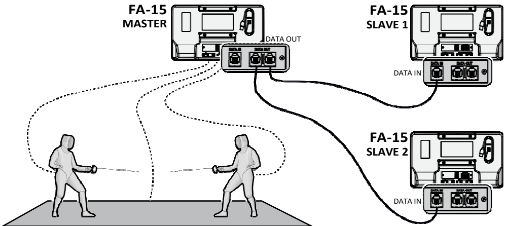
6. ábra Eszközök MASTER - SLAVE üzemmódban kábeles csatlakozással
