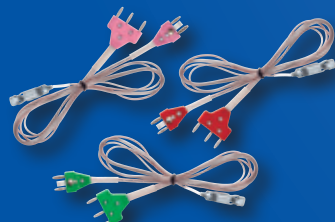
37631/T2 Foil/sabre body wire TRANSPARENT colored Transzparens tőr/kard testvezeték, színes
